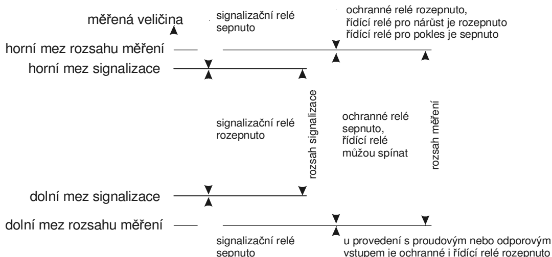
obr. III.3 – zobrazení rozsahu měření a rozsahu signalizace
